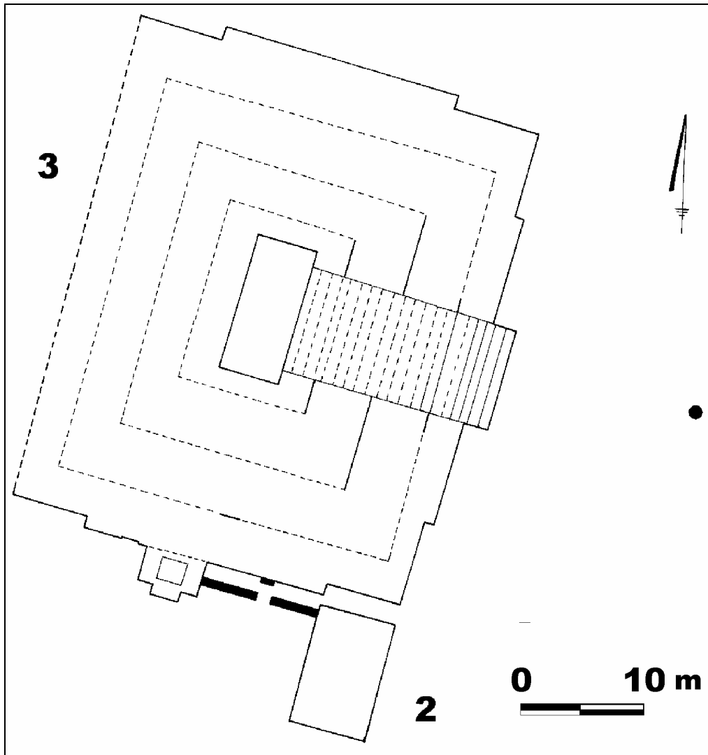
Figura 3 Planta específica de la Pirámide Oeste de la Plaza Norte
