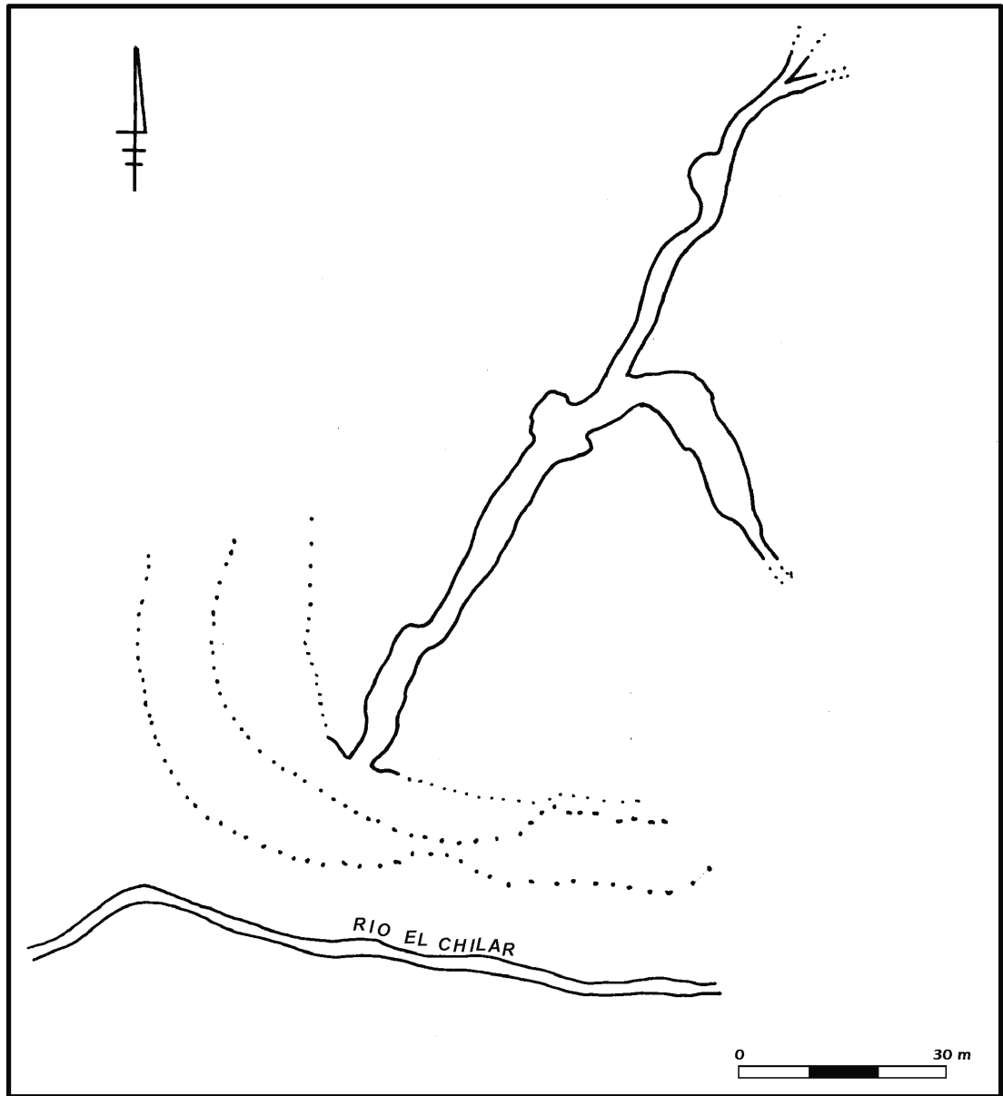
Figura 8 Planta de la Cueva de la Cerámica
