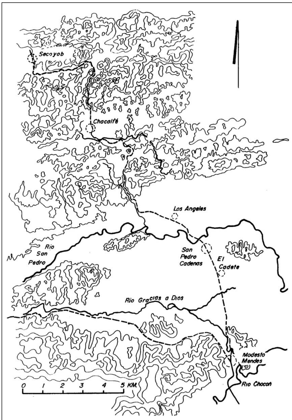
Figura 1 Zona reconocida entre los poblados de Secoyob y Modesto Méndez, Municipio de San Luis
