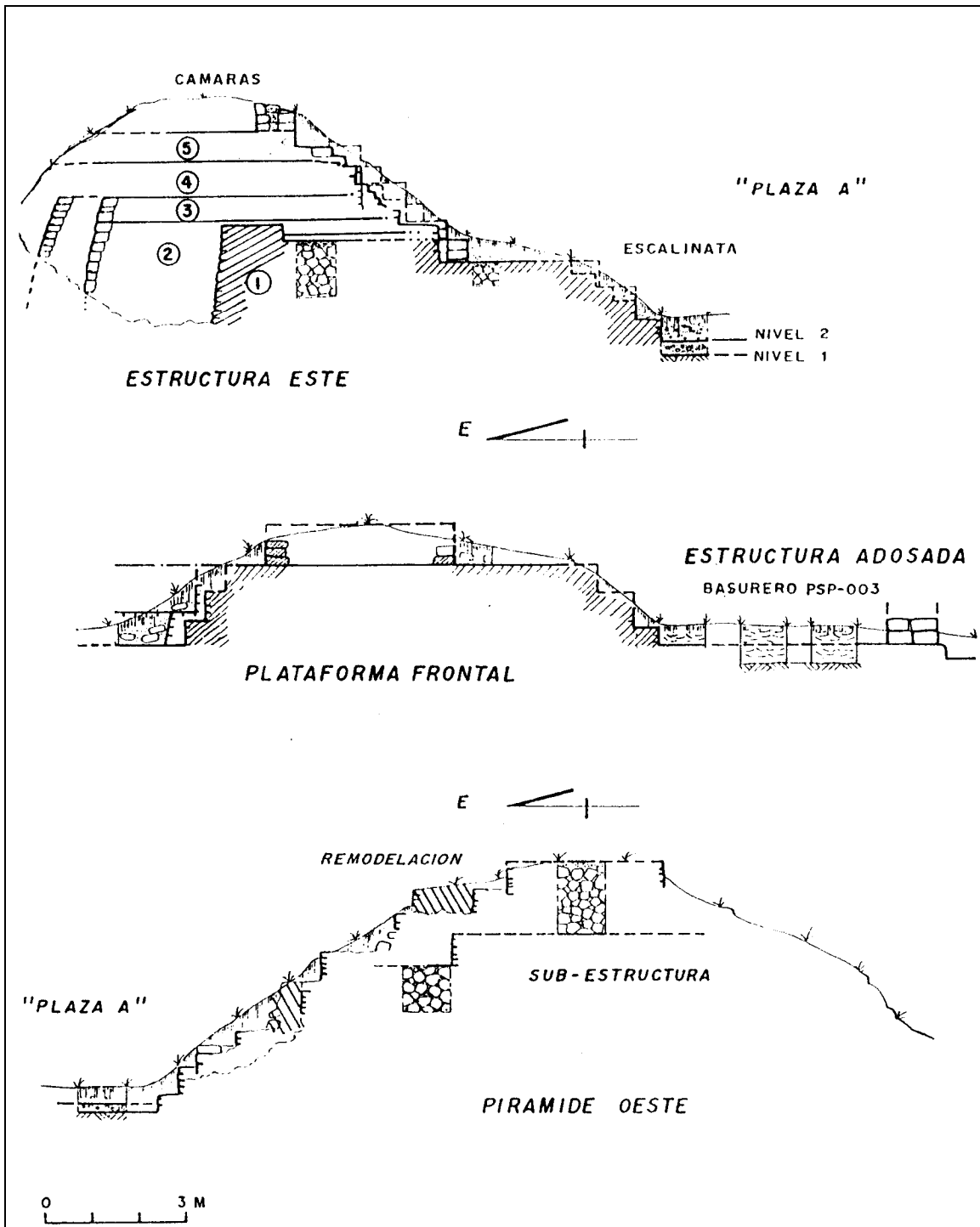
Figura 5 Corte este-oeste de la Estructura Este y el recinto en que se localizó el Depósito de Cerámica 3; corte este-oeste de la Pirámide Oeste
