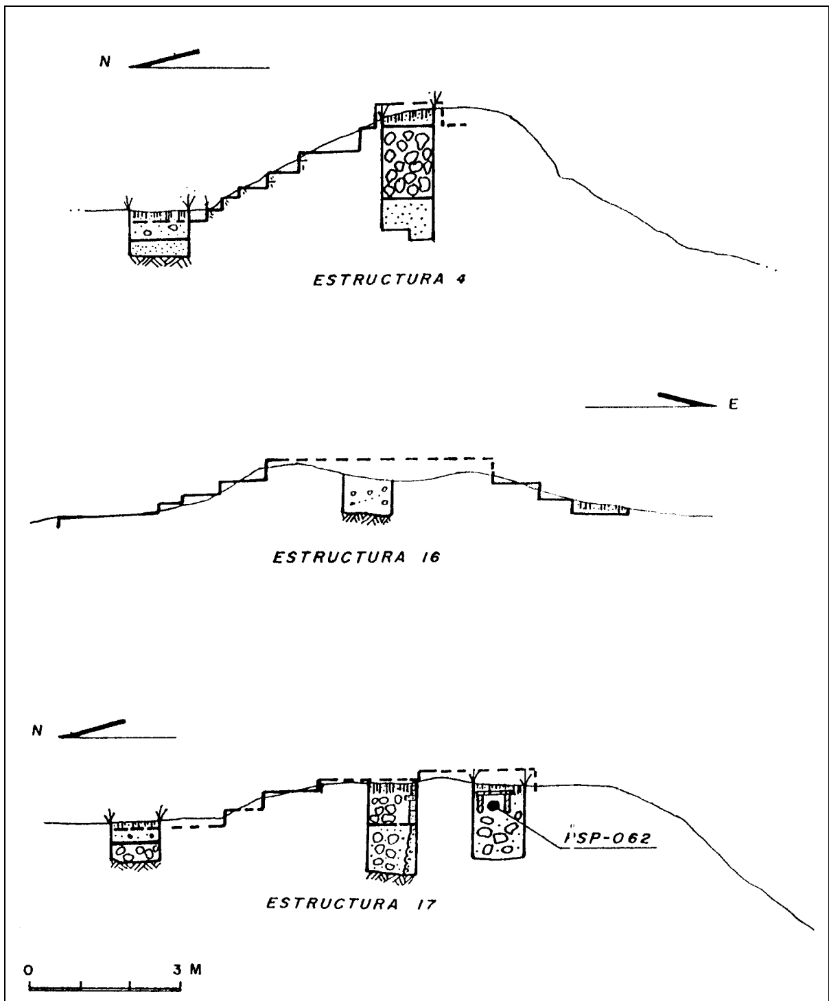
Figura 7 Cortes de las Estructuras 4 (Plaza A), 16 y 17 (Plaza D)
