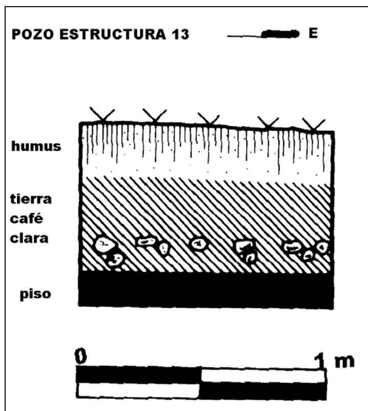
Figura 6 Pozo en el Grupo 14
